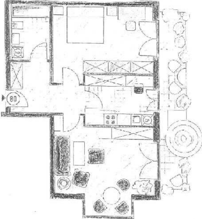
Grundriss Wohnung 80
